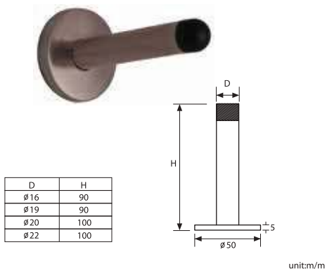
LOKRITE F01-022 HALF DOME DOOR STOP (10-S1-331) 152G-F01-02215
