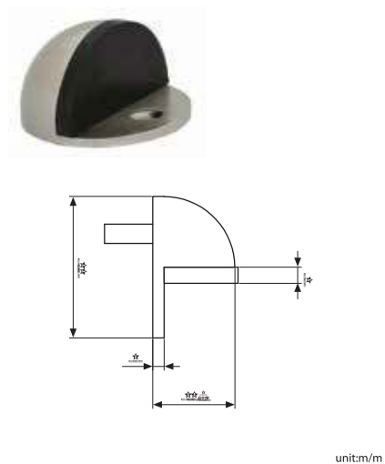
LOKRITE F01-022 HALF DOME DOOR STOP (10-S1-331) 152G-F01-02215
