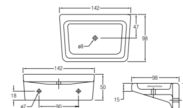
TOILET ROLL HOLDER WBSSTE000WW
