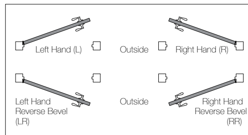
DOOR HANDING
